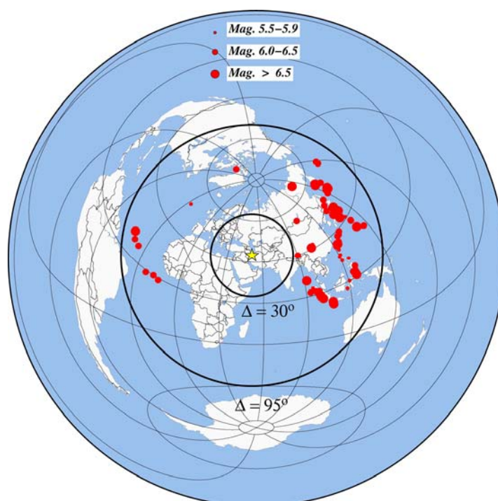
شکل ۲. رومرکز زمین‌لرزه‌های دورلرز استفاده شده در این تحقیق. زمین‌لرزه‌های دورلرز با بزرگی بیشتر از ۵/۵ در فواصل رومرکزی بین 30^\circ تا 90^\circ که با دایره‌های سرخ‌رنگ در ابعاد متفاوت، متناسب با بزرگی زلزله نشان داده شده است. دایره‌های سیاه‌رنگ فواصل رومرکزی بین 30^\circ تا 90^\circ را نشان می‌دهد. ستاره زرد رنگ مرکز نیم‌رخ مورد بررسی را نشان می‌دهد.
