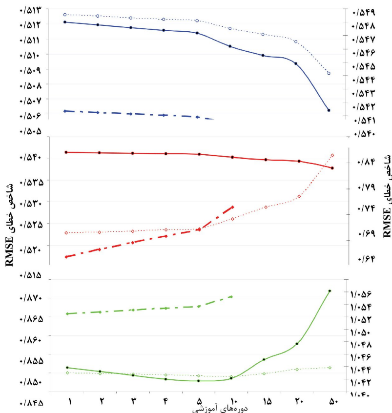
شکل ۸ نتایج پیش‌بینی سرعت باد در ارتفاع ۱۰ متری از زمین با استفاده از شبکه هوشمند (ترکیب ANFIS با یکی از روش‌های جست‌وجو): منحنی خط چین ضخیم برای ترکیب ANFIS با روش جست‌وجوی پیشرو، منحنی خط چین نازک برای ترکیب ANFIS با روش همبستگی متقابل و منحنی توپر برای ترکیب ANFIS با روش جست‌وجوی پسرو است. آموزش شبکه به روش ترکیبی که ترکیبی از روش کمترین مجذورات ۱ با روش گردایان نزولی پس‌انتشار خطا است. در این پیش‌بینی داده‌های توفان گونو برای آموزش، یمین برای آزمون و نرجس برای اعتبارسنجی به کار رفته است. مقادیر عرضه شده در سمت راست محور قائم مربوط به شبکه هوشمندی است که از ترکیب ANFIS با روش جست‌وجوی پسرو ساخته شده است.
