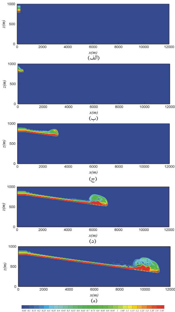
شکل ۵. تحول زمانی میدان شوری روی سطح شیب‌دار به روش مرتبه دوم مرکزی با اختلاف شوری \Delta S = 1.5 \text{ psu} برحسب ساعت، (الف) t = 0 \text{ h} ، (ب) t = 0.125 \text{ h} ، (ج) t = 1.5 \text{ h} ، (د) t = 3 \text{ h} ، (ه) t = 4.25 \text{ h} .
