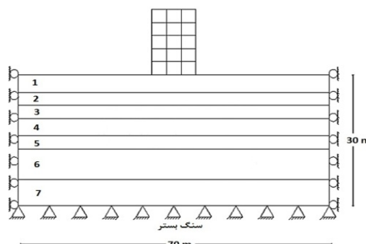
شکل ۳. نمونه مدل خاک و سازه برای خاک نوع ۳
