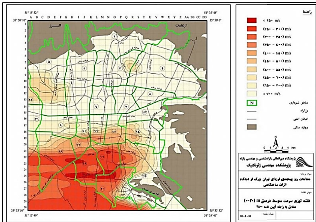
شکل ۱. نقشه پهنه‌بندی سرعت موج برشی برای تشخیص نوع ساختمانها در شهر تهران (جعفری و همکاران، ۱۳۸۲)
