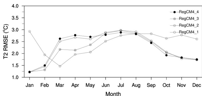
شکل ۳. میانگین ماهانه خطای ریشه میانگین مربعات دمای هوا در ارتفاع ۲ متری از سطح زمین در منطقه ایران برای چهار شبیه‌سازی مختلف انجام‌شده با RegCM4 در سال ۲۰۱۰. پارامترسازی‌های فیزیکی به کار رفته در چهار شبیه‌سازی مختلف در جدول ۱ آورده شده‌اند.
