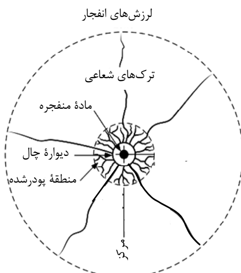
شکل ۳. مقطع چال انفجار و مناطق پنج‌گانه اطراف آن براساس پیشنهاد ایورسن و همکاران (۲۰۰۸).
