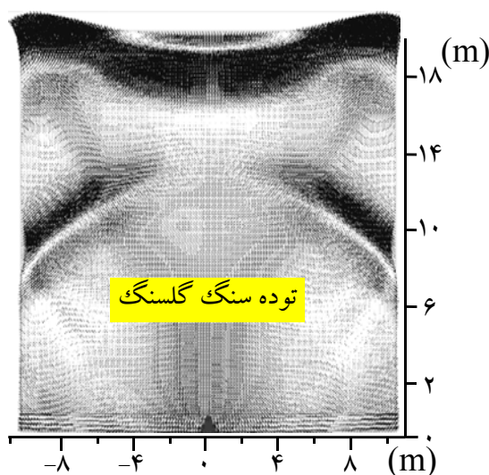
شکل ۱۰. بازتاب جبهه موج فشاری ناشی از انفجار از سطح آزاد در فاصله ۲۰ متری از مرکز انفجار پس از ۹/۲ میلی‌ثانیه.
