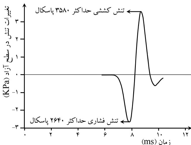
شکل ۱۱. تغییرات تنش فشاری به کششی در اثر بازتاب از سطح آزاد در فاصله ۲۰ متری از مرکز انفجار.
