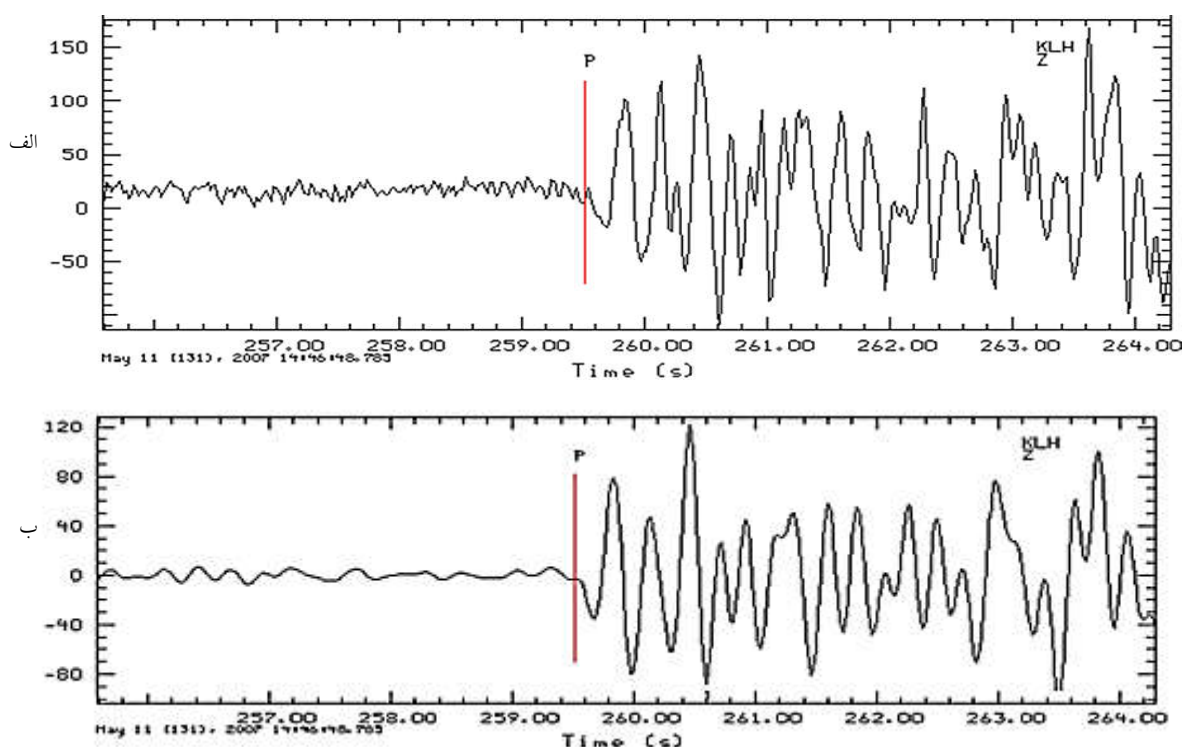
شکل ۲. بررسی شکل موج ثبت شده در ایستگاه کلاه‌رود، مربوط به رویداد یازده ماهه سال ۲۰۰۷ با بزرگای M_{\text{b}} 3/1 و فاصله رومرکزی ۱۰۵/۷ کیلومتر. (الف) شکل موج قبل از اعمال فیلتر، (ب) شکل موج بعد از اعمال فیلتر. استفاده از فیلتر علاوه بر افزایش نسبت سیگنال به نوفه در نگاشت لرزه‌ای، تغییری در قطبش اولین رسید موج P ایجاد نمی‌کند.
