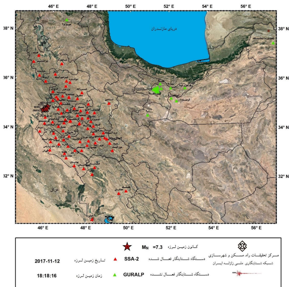
شکل ۱. نقشه ایستگاه‌های ثبت‌کننده زمین‌لرزه (مثلاً) به همراه رومرکزهایی که مراکز معتبر بین‌المللی (ستاره) گزارش کرده‌اند.
