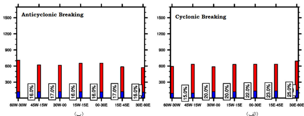
شکل ۱. تعداد شکست امواج در حالت‌های (الف) چرخندی و (ب) واپرخندی. میله‌های قرمز تعداد شکست امواج ( |i(\lambda, t)| > 1 ) و میله‌های آبی تعداد شکست متوسط و قوی امواج ( |i(\lambda, t)| > 2 ) را برای حالت‌های چرخندی و واپرخندی در هفت منطقه از غرب اقیانوس اطلس تا غرب آسیا (۶۰W-۶۰E) نشان می‌دهند. عدد کنار هر میله، نسبت تعداد شکست‌های متوسط و قوی به تعداد کل شکست‌ها برحسب درصد است.
