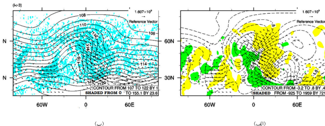
شکل ۶. (الف) بی‌هنجاری ارتفاع ژئوپتانسیل (۱۰۰ gpm، پربندها) در تراز ۲۰۰ hPa، همگرایی (ناحیه سبز، مقادیر منفی) و واگرایی (ناحیه زرد، مقادیر مثبت) شار فعالیت موج ( m/s^2 ) در لایه ۱۵۰-۳۰۰ hPa (ب) ارتفاع ژئوپتانسیل (۱۰۰ gpm، پربندها)، فعالیت موج ( m/s ، ناحیه آبی) و شار فعالیت موج ( m/s^2 ) بردارها) در لایه ۱۵۰-۳۰۰ hPa در شکست و اچرخندی امواج، حدود مقادیر شار فعالیت موج، همگرایی و واگرایی برای رنگ‌های آبی، زرد و سبز به ترتیب m/s ۰-۱۵۵، m/s^2 ۰-۰۰/۶ و m/s^2 ۰-۳/۲۰ است.
