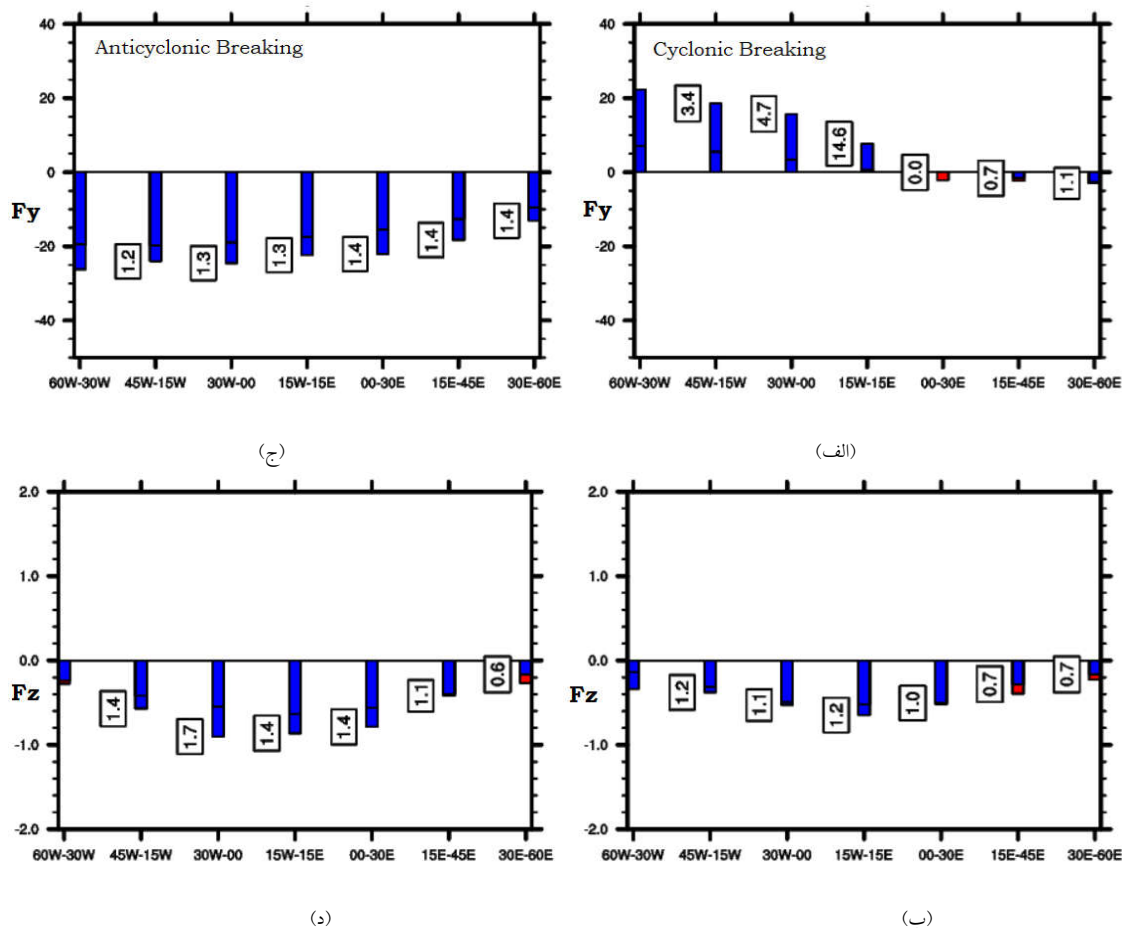
شکل ۱۰. میانگین شار (الف) قطب‌سوی فعالیت موجی ( 1 \times 10^{11} \text{ m}^2/\text{s}^2 )، در عرض 40^\circ\text{N} و (ب) پایین‌سوی فعالیت موجی ( 1 \times 10^{11} \text{ m}^2/\text{s}^2 ) در تراز ۲۰۰ hPa، برای شکست چرخندی (آبی) و متوسط (قرمز) یک موج برای هفت ناحیه از غرب اقیانوس اطلس تا غرب آسیا ( 60^\circ\text{E} – 60^\circ\text{W} ). عدد کنار هر میله نسبت این دو مقدار را در هر منطقه مشخص می‌کند. نمودارهای (ج) و (د) مشابه نمودارهای (الف) و (ب) ولی برای شکست و اچرخندی هستند.
