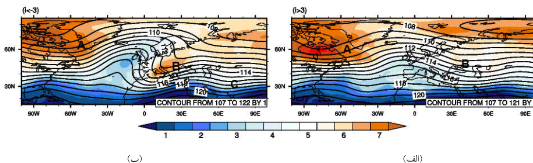
شکل ۲. میانگین ارتفاع ژئوپتانسیل (۱۰۰ gpm، پریندها) در تراز ۲۰۰ hPa و تاوایی پتانسیلی (PVU، ناحیه رنگی) در لایه ۳۰۰-۱۵۰ hPa برای (الف) شکست چرخندی و (ب) شکست و اچرخندی امواج روی مدیترانه و اروپا.
