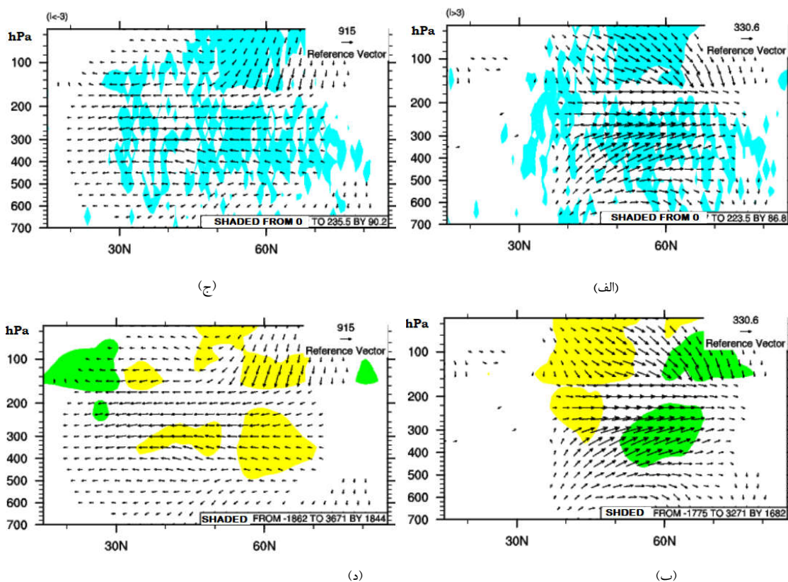
شکل ۸. میانگین مداری شار فعالیت امواج ( 1 \times 10^6 \text{ m}^2/\text{s}^2 ، بردارها)، فعالیت امواج ( \text{m/s} ، ناحیه آبی‌رنگ) برای (الف) شکست چرخندی و (ج) شکست واپرخندی و همگرایی (ناحیه سبز، منفی) و واگرایی (ناحیه زرد، مثبت) شار فعالیت امواج ( \text{m/s}^2 ) برای (ب) شکست چرخندی و (د) شکست واپرخندی. مقادیر در پوشش‌سپهر زیرین ( 100\text{--}50 \text{ hPa} ) در 10^\circ ضرب شده است. در شکست واپرخندی (ج و د)، حدود مقادیر برای رنگ‌های آبی، زرد و سبز به ترتیب 0\text{--}235 \text{ m/s} ، 0\text{--}3671 \text{ m/s}^2 و -1662\text{--}3671 \text{ m/s}^2 است. در شکست چرخندی (الف و ب)، حدود مقادیر برای رنگ‌های آبی، زرد و سبز به ترتیب 0\text{--}223 \text{ m/s} ، -1775\text{--}3271 \text{ m/s}^2 و -1682\text{--}3271 \text{ m/s}^2 است.
