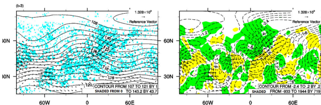
شکل ۷. مشابه شکل ۶ اما برای شکست چرخندی امواج. حدود مقادیر برای رنگ‌های آبی، زرد و سبز به ترتیب m/s ۰-۱۴۳، m/s^2 ۰-۱۹۴۴ و m/s^2 ۰-۹۳۳ است.
