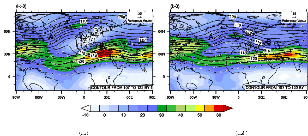
شکل ۴. میانگین ارتفاع ژئوپتانسیل (۱۰۰ gpm)، پربندها، میدان باد (متر بر ثانیه، بردارها) و جت (ناحیه رنگی) در تراز ۲۰۰ hPa برای (الف) شکست چرخندی (ب) شکست واچرخندی امواج.
