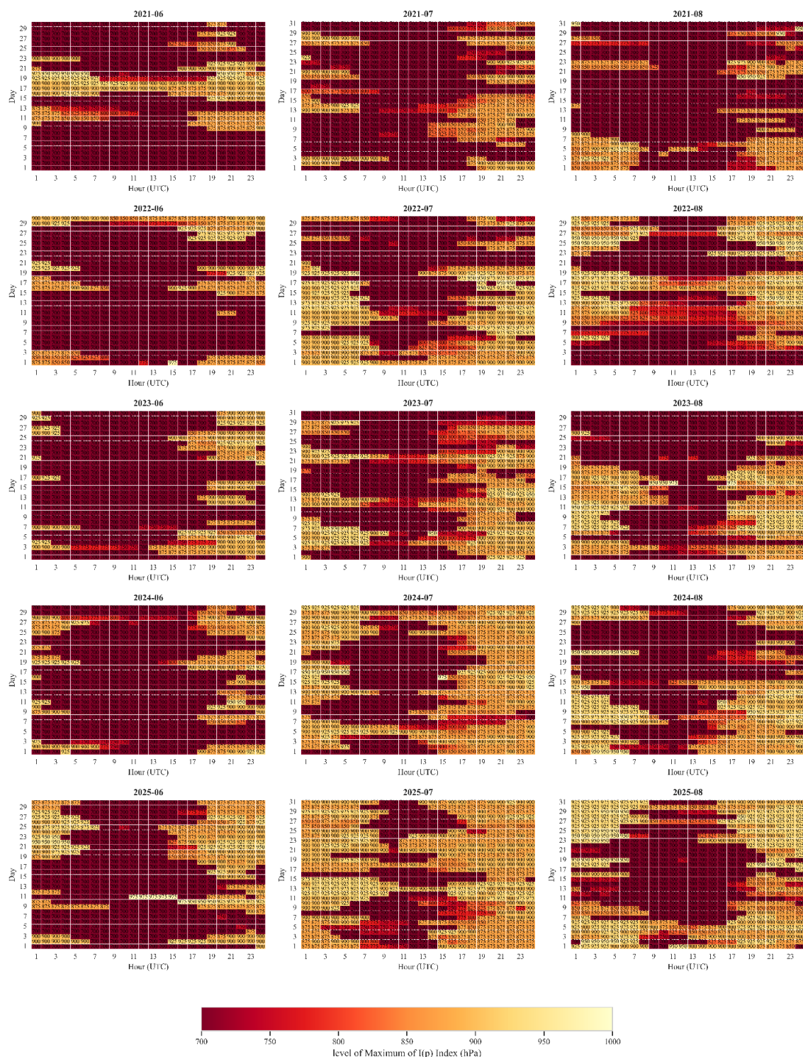
شکل ۲. نقشه‌های حرارتی روز-ساعت تراز بیشینه I(p) برای ماه‌های ژوئن، ژوئیه و اوت در دوره‌ی ۲۰۲۱-۲۰۲۵ بر اساس داده‌های ERA5 (دامنه‌ی فشار: سطح زمین تا ۷۰۰ هکتوپاسکال).
