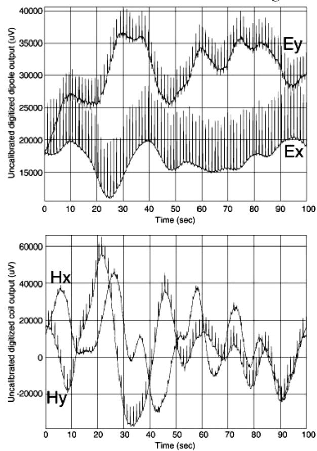
شکل ۶. نوفه‌های ولتاژ بالا با دوره تناوبی بسیار کوتاه ناشی از یک حفاظ نرده‌ای الکتریکی که بر سیگنال‌های اصلی میدان‌های EM قرار گرفته‌اند (اشتایگپول و همکاران، ۲۰۰۹).
