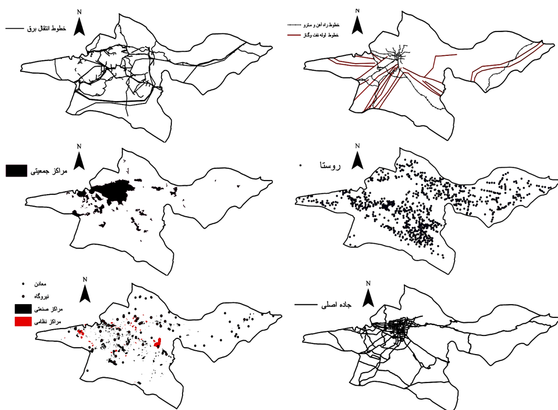
شکل ۹. لایه‌های اطلاعاتی مربوط به توزیع مکانی مولدهای مصنوعی نوفه‌های EM در محدوده استان تهران.
