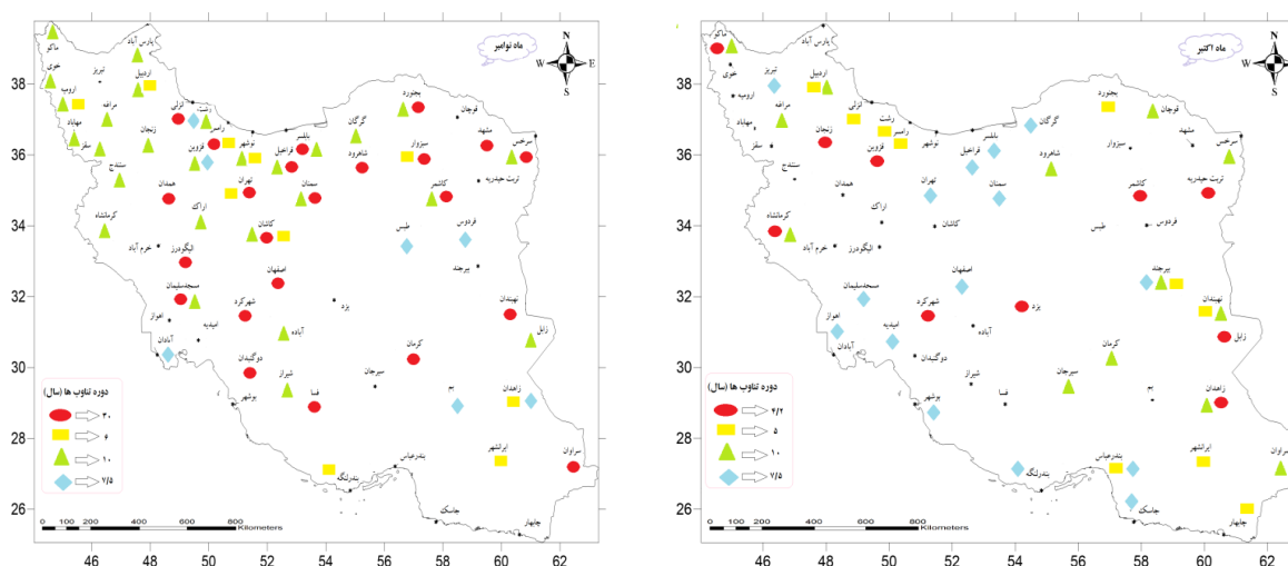
شکل ۲. توزیع مکانی دوره‌های تناوبی ایستگاه‌ها برای ماه‌های اکتبر و نوامبر.
