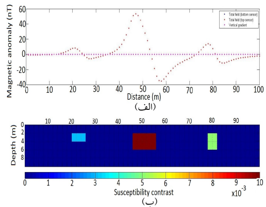
شکل ۱. (الف) تغییرات شدت میدان مغناطیسی (نانوتسلا) در راستای پروفیل (فاصله برحسب متر)، نقاط قرمز نشان‌دهنده میدان کل و نقاط صورتی گرادیان قائم (ب) مدل مصنوعی در نظر گرفته شده (محور افقی تبارین پذیرفتاری و محور قائم عمق بر حسب متر).
