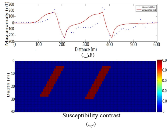
شکل ۸. (الف) تغییرات شدت میدان مغناطیسی در راستای پروفیل شماره ۷ (نقاط آبی نشان دهنده میدان کل مشاهده شده و خط قرمز میدان کل محاسبه شده، (ب) مدل اولیه حاصل از مدل‌سازی پیشرو برای وارون‌سازی پروفیل شماره ۷.
