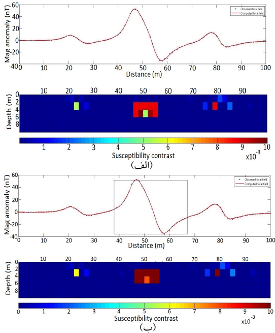
شکل ۲. نتایج حاصل از وارون‌سازی مدل مصنوعی (نقاط آبی میدان کل مشاهده شده و خط قرمز نشان‌دهنده میدان کل و بدون کاربرد روش ماسک سیگنال و (ب) با کاربرد روش ماسک سیگنال.
