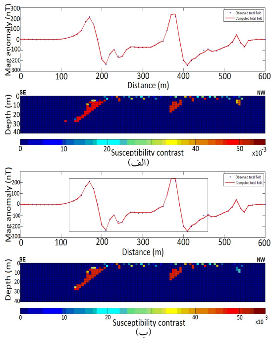
شکل ۷. نتایج حاصل از فرایند وارون‌سازی پروفیل شماره ۷، نقاط آبی میدان کل مشاهده شده و خط قرمز میدان کل محاسبه شده، (الف) بدون کاربرد روش ماسک سیگنال، (ب) همراه با کاربرد روش ماسک سیگنال.
