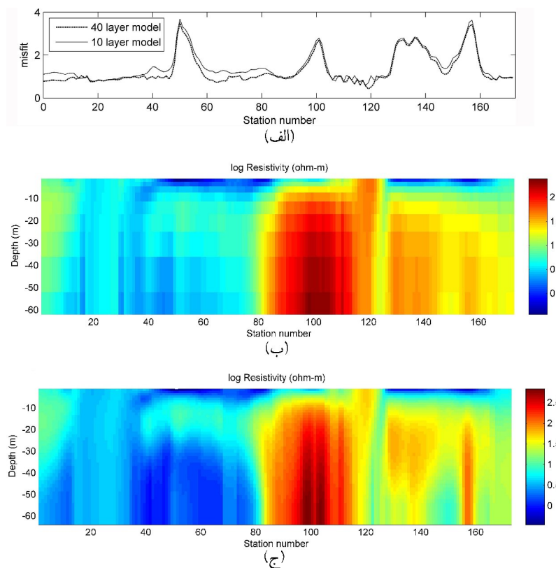
شکل ۶. پاسخ فرایند وارون‌سازی داده‌های واقعی. منحنی عدم برازش نرمال شده برای هر دو مدل در (الف) نمایش داده شده است، مدل مورد نظر در (ب) ۱۰ لایه و در (ج) ۴۰ لایه است. ضخامت لایه اول در هر دو مدل ۱ متر است. واضح است که هرچه تعداد لایه‌ها بیشتر باشد مدل بهتری به دست می‌آید.
