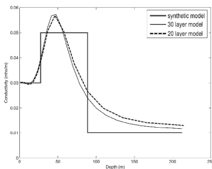
شکل ۵. اثر تعداد لایه‌ها بر پاسخ فرایند وارون‌سازی. در عمق پایین‌تر، مدل ۳۰ لایه مصنوعی را بهتر بازسازی کرده و می‌توان گفت هرچه تعداد لایه‌ها بیشتر باشند مدل بهتری به دست می‌آید.
