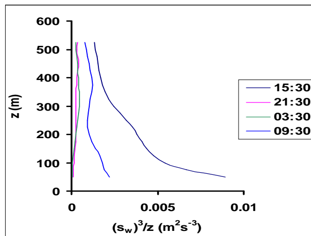
شکل ۵. نمایه قائم کمیت تلاطمی (s_w)^3/z (میانگین ساعتی از ۱۳ تا ۲۴ اوت ۲۰۰۲).
