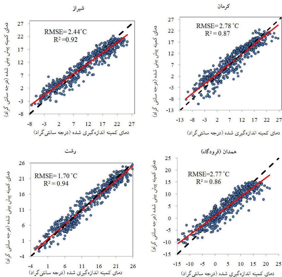
شکل ۲. مقایسه برازش مقادیر اندازه‌گیری شده و پیش‌بینی شده دمای کمینه در روز آتی توسط مدل رگرسیونی لیناگر در دوره سالانه.
