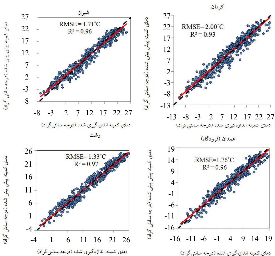
شکل ۴. مقایسه برازش مقادیر اندازه‌گیری شده و پیش‌بینی شده دمای کمینه در روز آتی توسط شبکه‌های عصبی مصنوعی منتخب با سه ورودی (دمای نقطه شبنم، بیشینه دما و رطوبت نسبی) در دوره سالانه.
