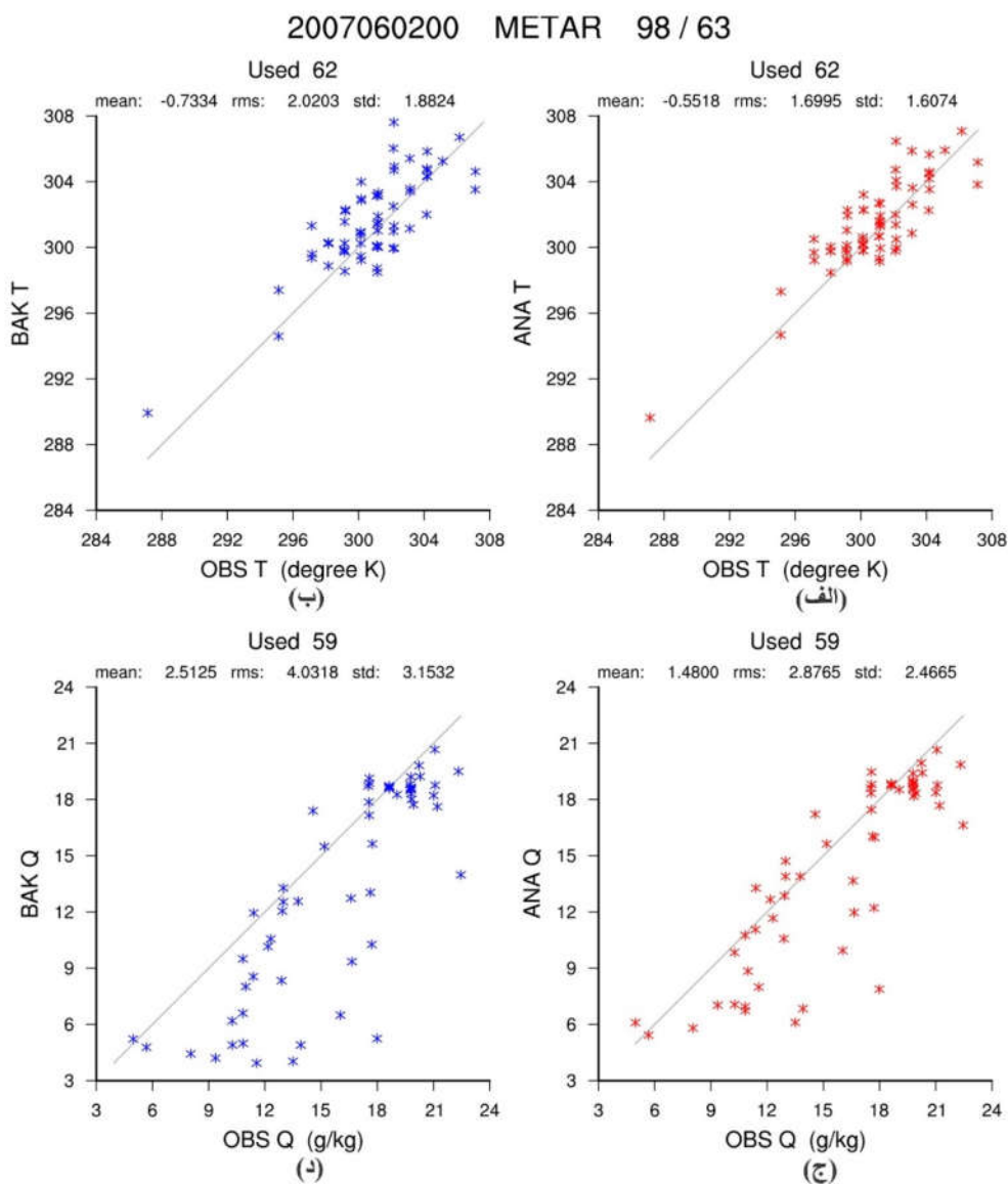
شکل ۵. پراکندگی داده‌های تحلیل‌شده و داده‌های حدس اولیه در مقایسه با داده‌های مشاهدات برای داده‌گویی داده‌های METAR/T و METAR/Q. محورهای افقی برای هر چهار شکل، معرف داده‌های مشاهدات و محورهای عمودی برای شکل‌های (الف) و (ج) به ترتیب معرف داده‌های تحلیل‌شده دما و رطوبت مطلق هستند. محورهای عمودی برای شکل‌های (ب) و (د)، معرف داده‌های حدس اولیه دما و رطوبت مطلق هستند. شکل‌ها بیانگر این هستند که پراکندگی داده‌ها در حالت تحلیل‌شده کاهش یافته است و به مشاهدات نزدیک‌تر می‌شود.
