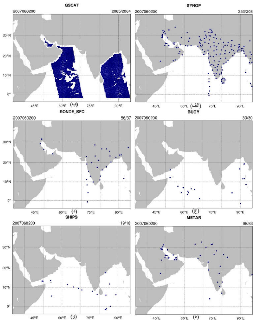
شکل ۴. توزیع مکانی داده‌های استفاده‌شده در انجام داده‌گواری برای محدوده اول (الف) داده‌های SYNOP (ب) داده‌های QSCAT (ج) داده‌های BUOY (د) داده‌های SONDE_SFC (ه) داده‌های METAR (و) داده‌های SHIPS. بیشترین داده‌ها مربوط به ماهواره QSCAT و کمترین داده‌ها مربوط به داده‌های جمع‌آوری‌شده با استفاده از کشتی‌ها (SHIPS) است. اعداد نوشته‌شده در بالای سمت راست هر شکل، به ترتیب مربوط به کل داده‌های موجود سنجنده و داده‌های استفاده‌شده سنجنده مورد نظر در انجام داده‌گواری است.
